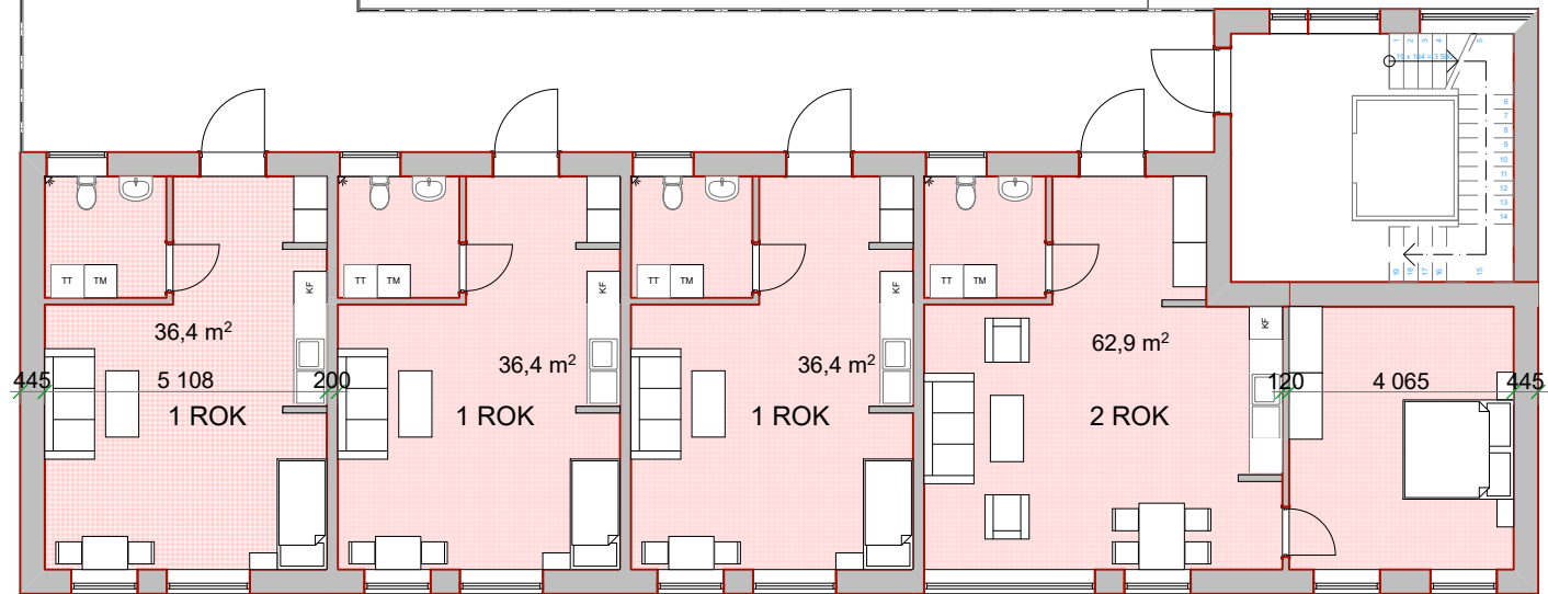
PLAN 2&3 SKALA 1:150 A3
